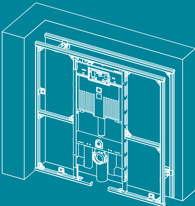
Vgradnja v sprednjo steno TECEprofil
