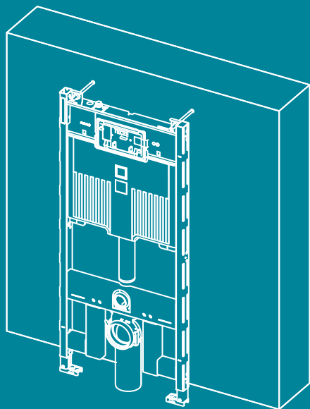
Vgradnja posamezne enote pred masivno steno
