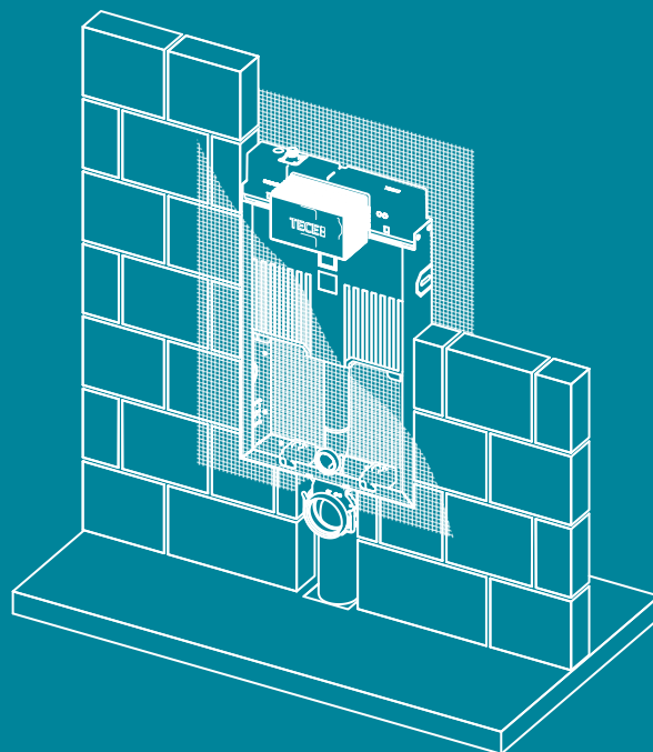
Ugradnja u predzid od opeke
