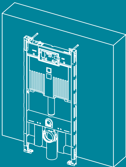
Ugradnja pojedinačnog modula ispred punog nosivog zida
