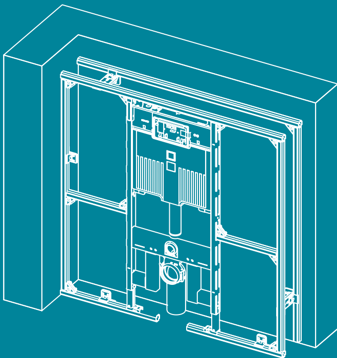
Ugradnja u TECEprofil predzid
