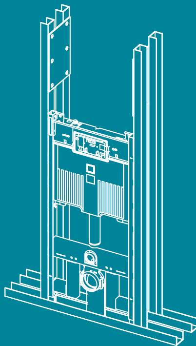
Ugradnja u metalne i drvene konstrukcije
