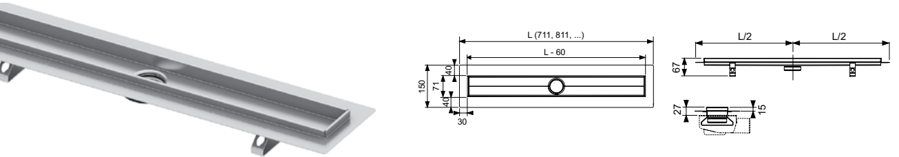
Canaletta lineare “Classic” in acciaio inox
