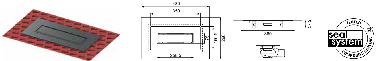
Set canaletta doccia per pavimenti continui, con inserto canaletta rivestibile
