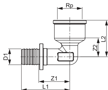
TECEflex - Gomito a 90° con manicotto filetto interno
