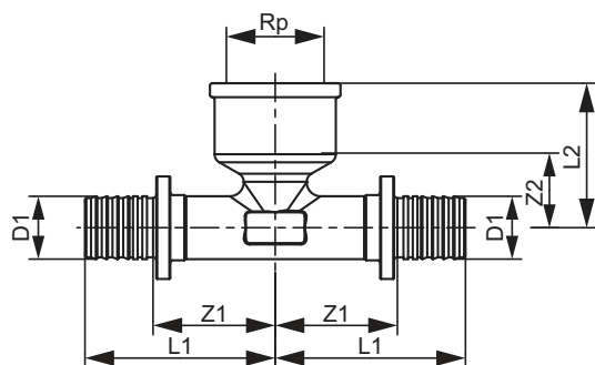
TECEflex - Raccordo a "T" con filetto interno
