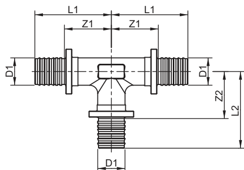
TECEflex - Raccordo a "T"
