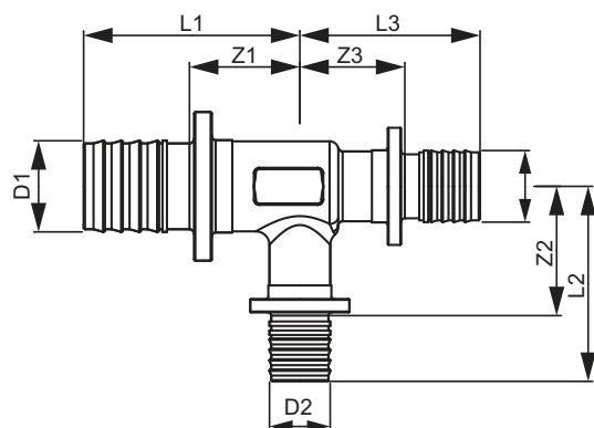
TECEflex - Raccordo a "T" ridotto
