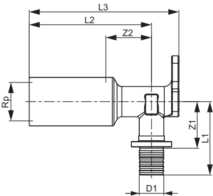
TECEflex - Terminale a parete, lungo
