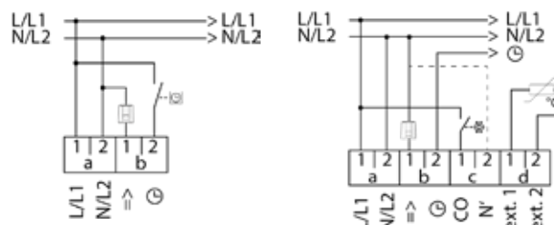
Schaltplan RT-D Standard
