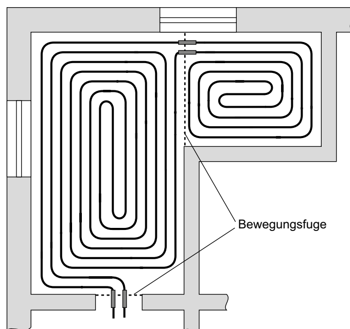
Position der Bewegungsfugen und Lage der Schutzrohre
