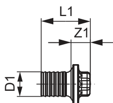
TECEflex zaślepka
