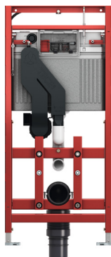
TECElux module 300
