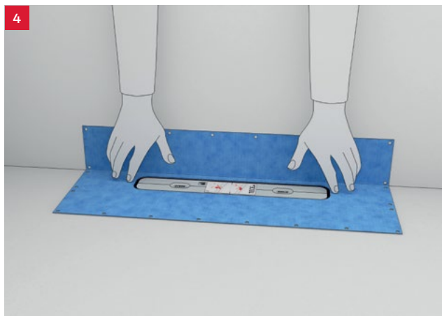
Montera tätskiktet Tryck fast den medföljande tätskiktsfolien i spåret runt avloppet. Arbeta in den i duschutrymmets tätskikt.
