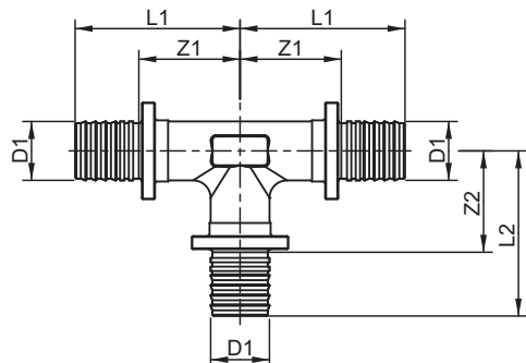
TECEflex trójnik 90°
