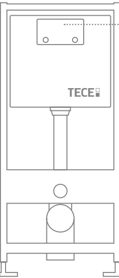
9240999 Заглушка Размер (ш x в x г): 220 x 170 x 2 мм Нержавеющая сталь, сатин
