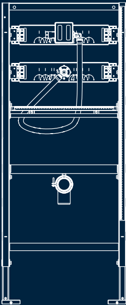
Застенный модуль TECE для писсуара с клапаном смыва U1
