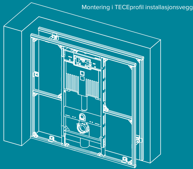
Montering i TECEprofil installasjonsvegg
