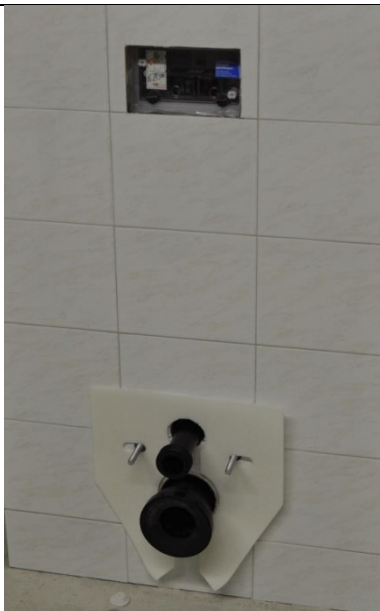
9. Etter at tettemassen har herdet, kan montasjen av porselent forberedes ved å sette skumplaten på plass. NB! Skumplaten skal monteres, da den sørger for dremsåpning i tillegg til støydemping.
