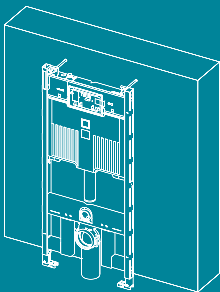
Individuele installatie van het inbouwframe voor een massieve ruwbouwmuur
