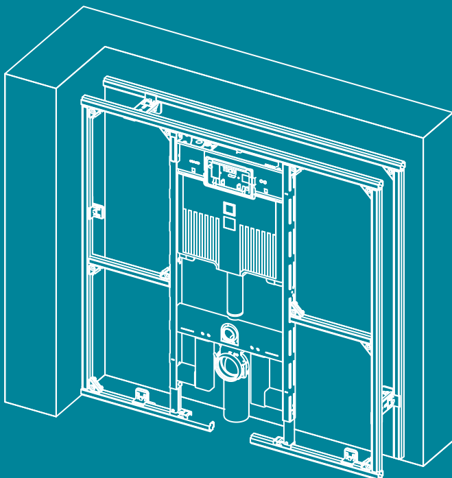
Installatie in een TECEprofil voorwand
