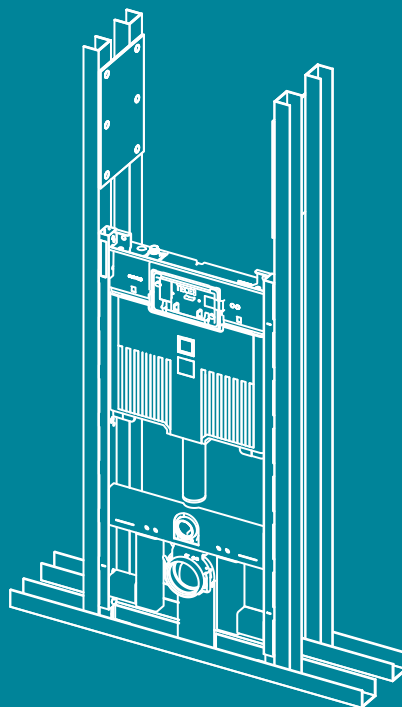
Installatie in metalen profielen en houtprofielwanden
