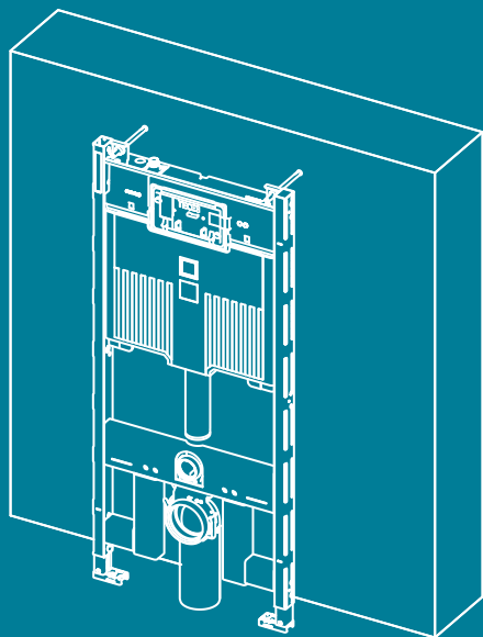
Instalación de módulo individual delante del armazón estructural de una pared maciza
