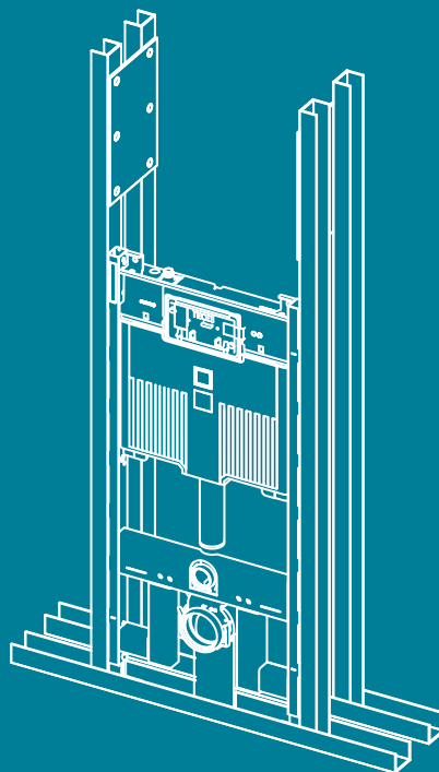
Instalación en perfiles metálicos y paredes de entramado de madera
