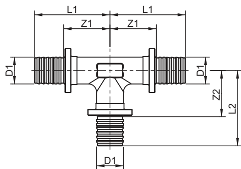
TECEflex T-stuk
