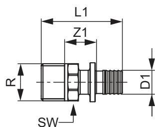
TECEflex väliskeermega liitmik
