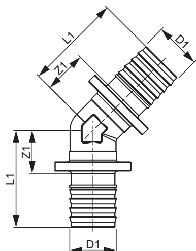
TECEflex 45° põlv
