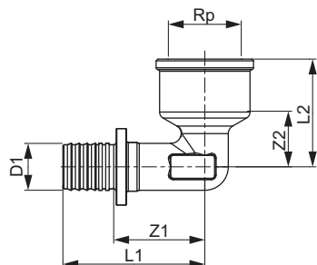
TECEflex sisekeermega põlv
