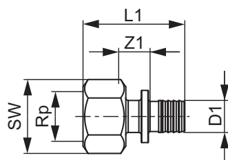
TECEflex sisekeermega liitmik
