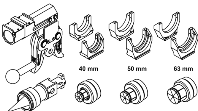
Urządzenie zaciskowe PMA 40 63 TECEflex
