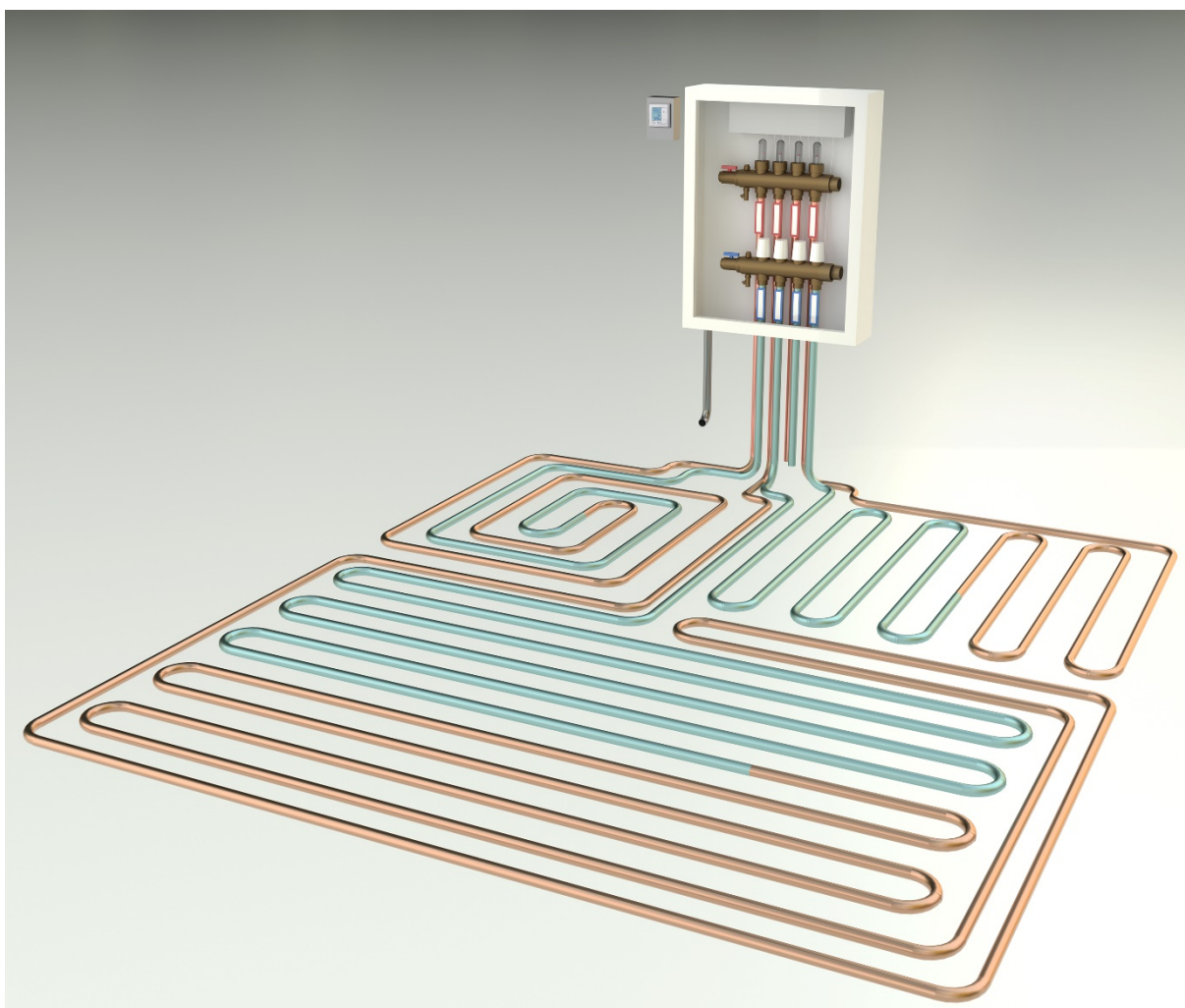
Figur 1 – Illustrasjon av vannbåren gulvvarme med rør, fordelerskap og termostad.
