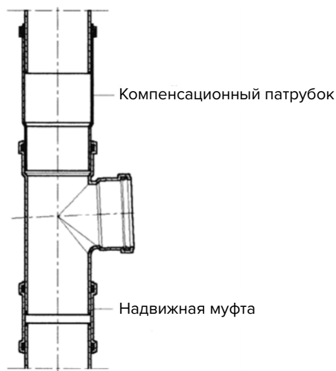
Монтаж тройника с использованием компенсационного патрубка и надвижной муфты
