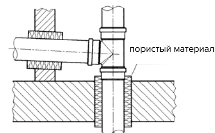
Прокладка труб через стены и потолочные перекрытия
