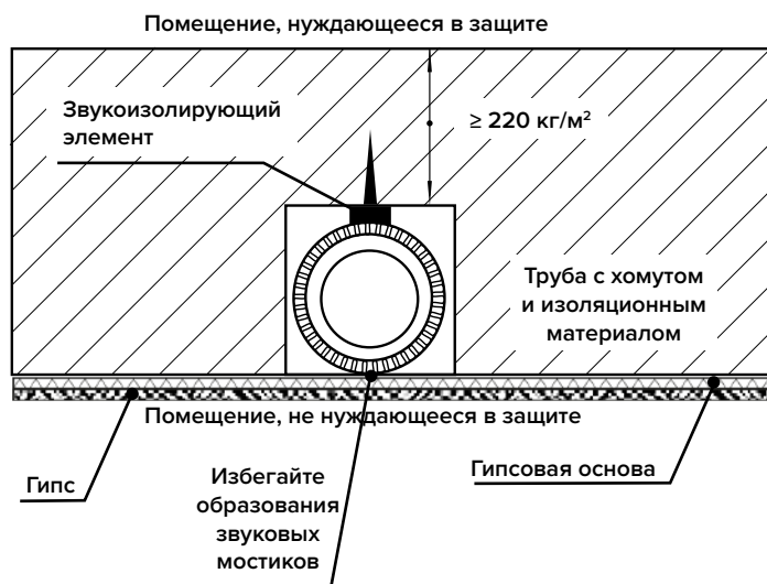
Исключение образования мостиков ударного шума
