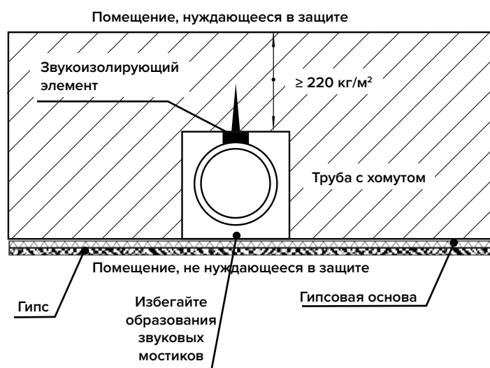
Традиционный метод прокладывания
