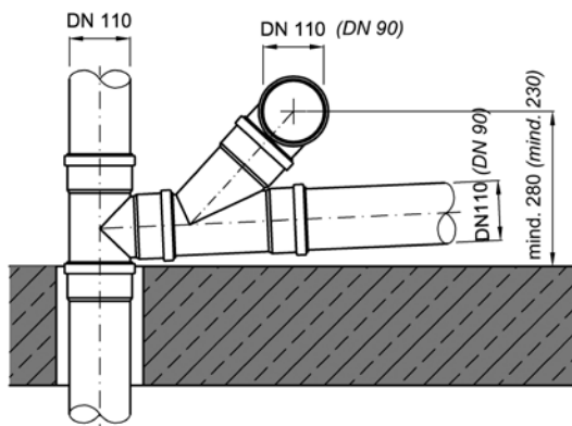
Монтаж со стандартным тройником
