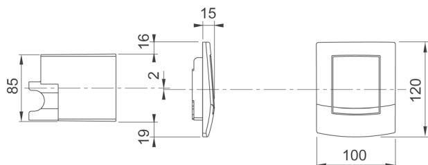
Urinal betjeningsplate og beskyttelsesdeksel for vertikal fugeretning
