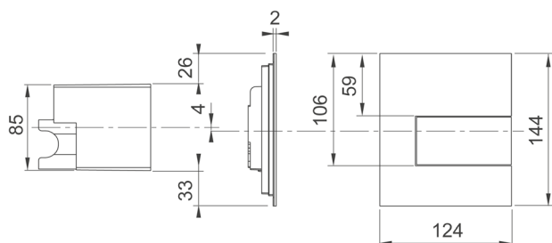
Urinal betjeningsplate og beskyttelsesdeksel for vertikal fugeretning
