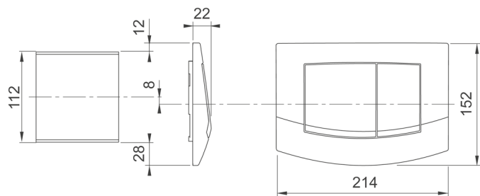
Dimensjoner WC-betjeningsplate og beskyttelsesdeksel for vertikal fugeretning
