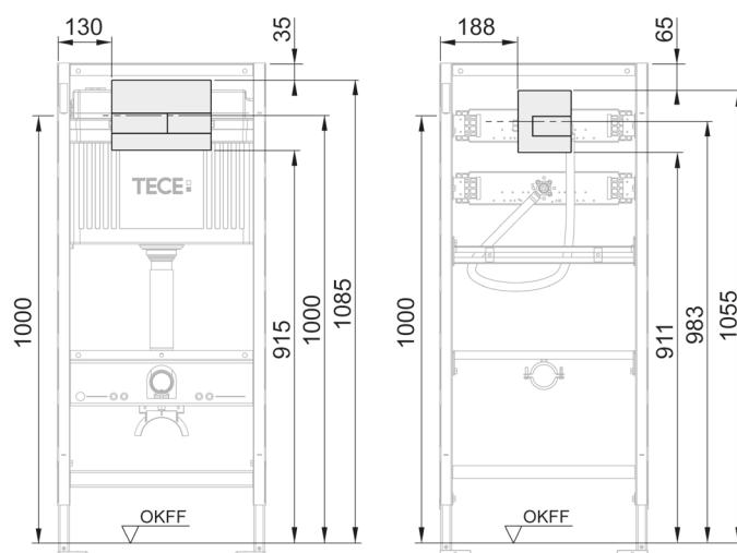
WC-betjeningsplate (venstre) og Urinal betjeningsplate (høyre) Modul 1120 mm
