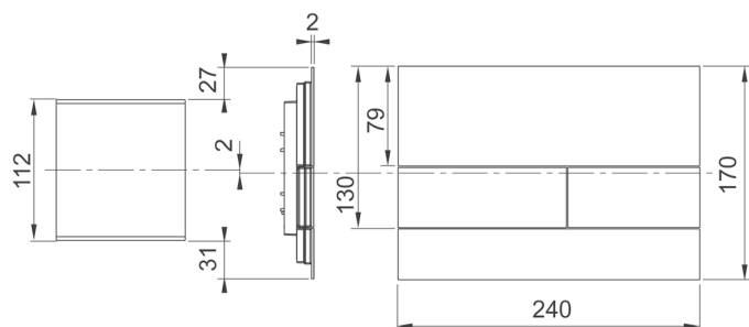
Dimensjoner WC-betjeningsplate og beskyttelsesdeksel for vertikal fugeretning
