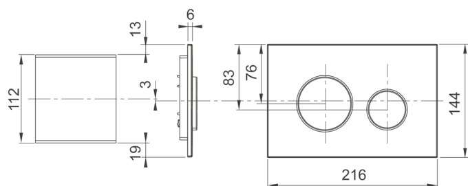
Dimensjoner WC-betjeningsplate og beskyttelsesdeksel for vertikal fugeretning
