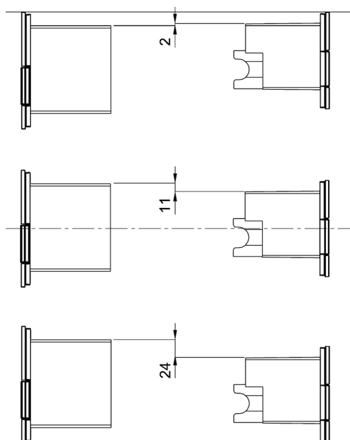
Urinal betjeningsplate og beskyttelsesdeksel for vertikal fugeretning
