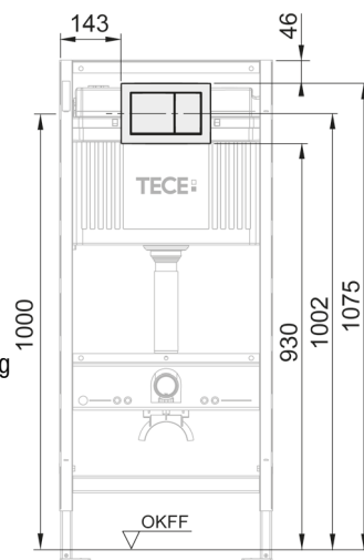
WC-betjeningsplate Modul 1120 mm
