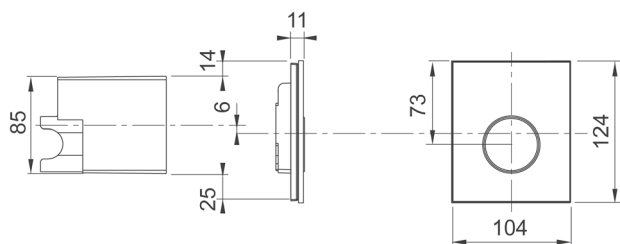
Urinal betjeningsplate og beskyttelsesdeksel for vertikal fugeretning
