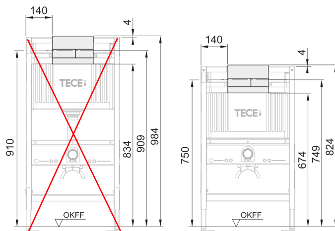
WC-betjeningsplate Modul 820 mm (980 mm leveres ikke i Norge)
