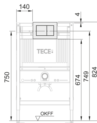
WC-betjeningsplate Modul 820 mm (980 mm leveres ikke i Norge)
