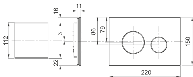
Dimensjoner WC-betjeningsplate og beskyttelsesdeksel for vertikal fugeretning
