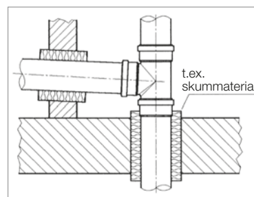
Vägg- och takgenomföringar (FIGUR 26)
