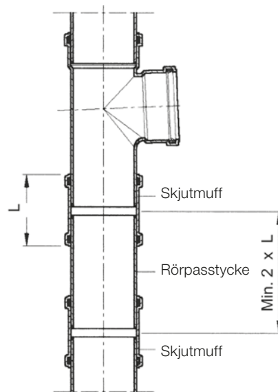
Inbyggnad av grenrör med 2 skjutmuffar (FIGUR 32)
