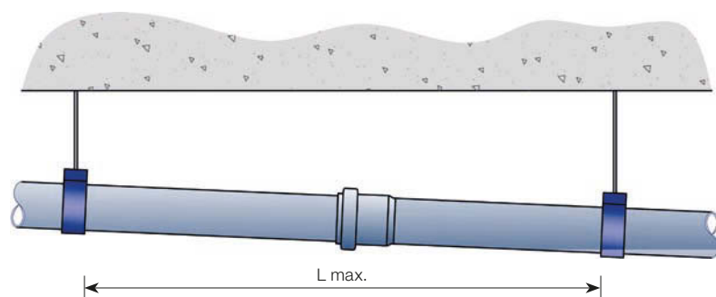
Vågrät ledningsdragning (FIGUR 22)
