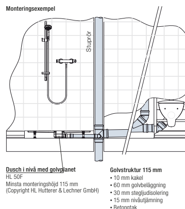
Installationsexempel dubbelt hörngrenrör (FIGUR 34)
