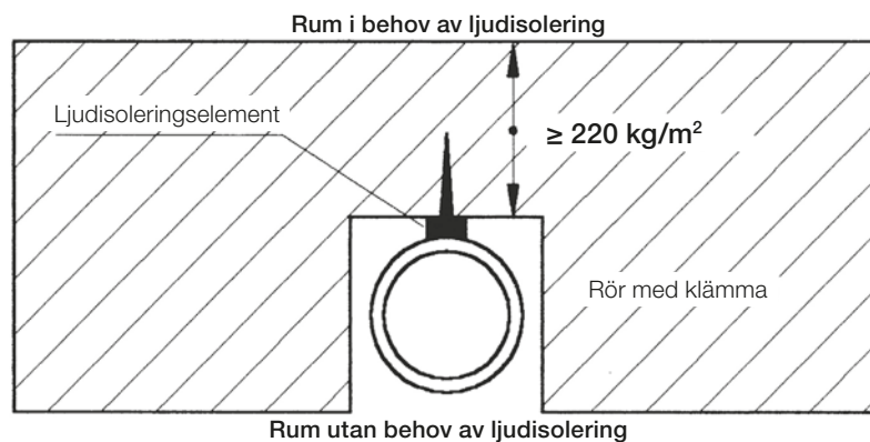
Montering med ljudisoleringsselement (FIGUR 27)
