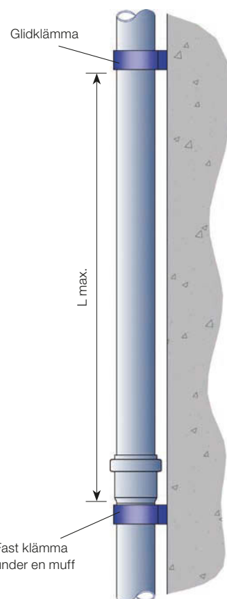
Lodrät ledningsdragning (FIGUR 23)
