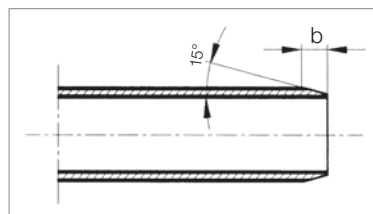
Fasning under en vinkel på ca 15° (FIGUR 21)
