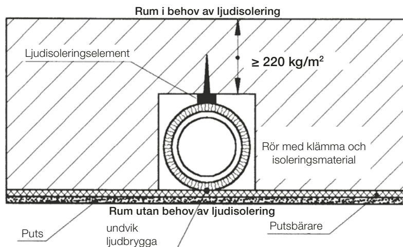
Förebyggande av bryggor för strukturburet buller (FIGUR 29)
