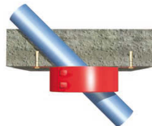
Tak specialtillämpning "sned montering 45°" (FIGUR 62)
