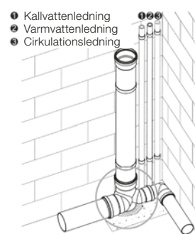
Installationsexempel kombinationsgrenrör (FIGUR 35)
