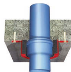
Tak specialtillämpning "montering över muff" (FIGUR 63)
