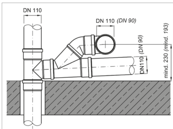
Monteringssituation med parallellgrenrör 45° (FIGUR 55)
