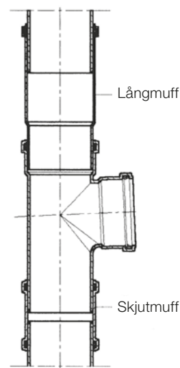
Inbyggnad av grenrör med lång- och skjut- muff (FIGUR 33)
