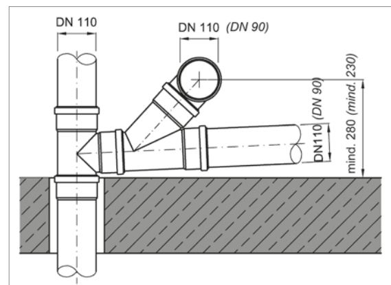
Monteringssituation med standardgrenrör (FIGUR 56)
