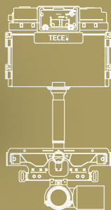
Anschlusseinheiten für WC, Waschtisch oder Urinal, ohne Modulrahmen zur direkten Montage im TECEprofil Tragwerk
