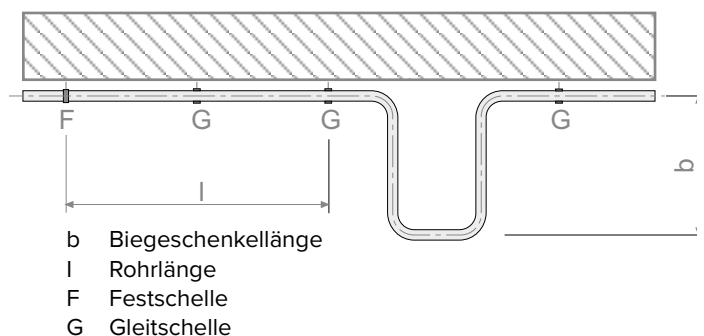
Abfangen der thermischen Längenausdehnung in einer Dehnungsschleife
