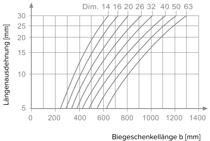
Biegeschenkelänge für TECElogo Rohre
