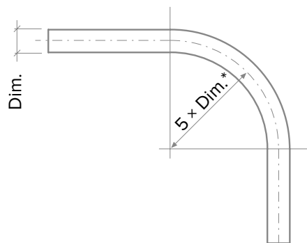
Minimaler Biegeradius der TECEflex Verbundrohre
