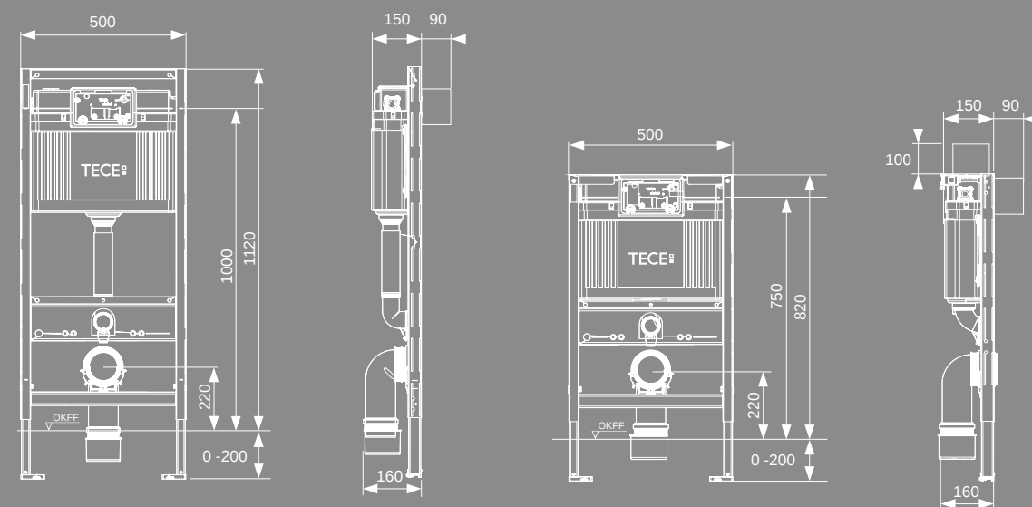
TECEprofil, höjd 1120 mm, frontaktivering RSK nr: 7926156 RSK nr: 7926157 (med SafetyBag)
