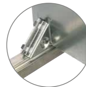
Einfache Reihenmontage mehrerer TECEbox WC-Module mit TECEprofil Rohr und Eckverbinder.
