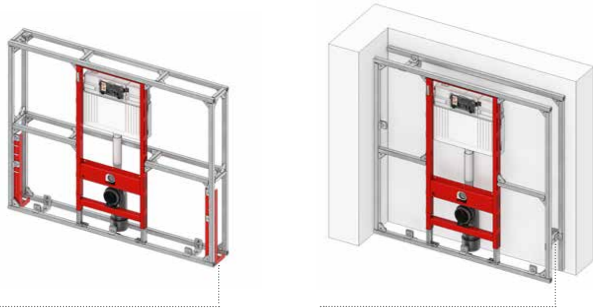
Einbau in freistehender TECEprofil Wand TECEprofil Stützfüße zur Aussteifung von freistehenden TECEprofil Tragwerken.
