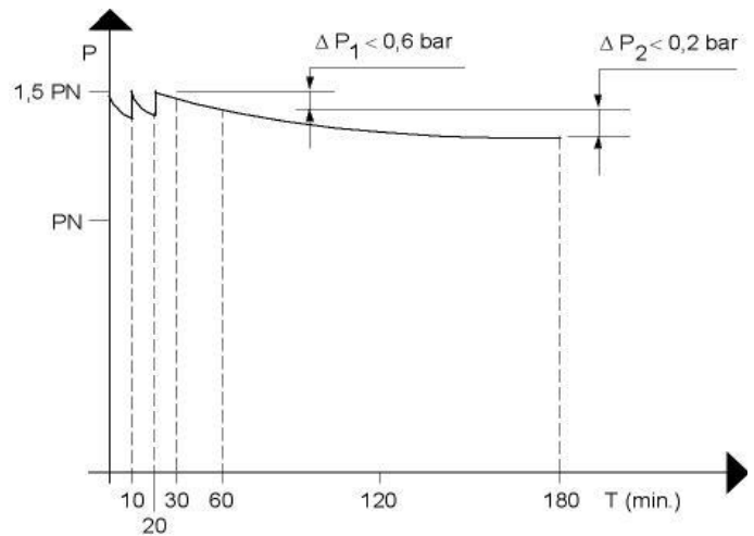
Figuur 1 - Dichtheidscontrole
