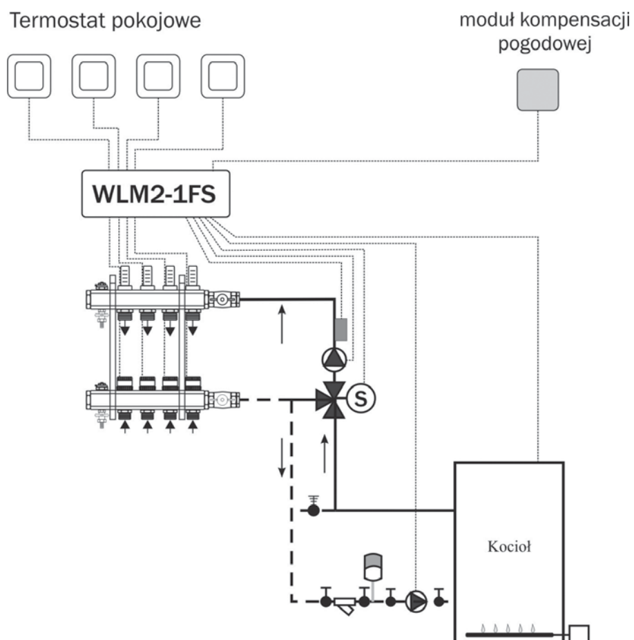
Sterowanie z wykorzystaniem kompensacji pogodowej z wykorzystaniem zaworu 3-drogowego
