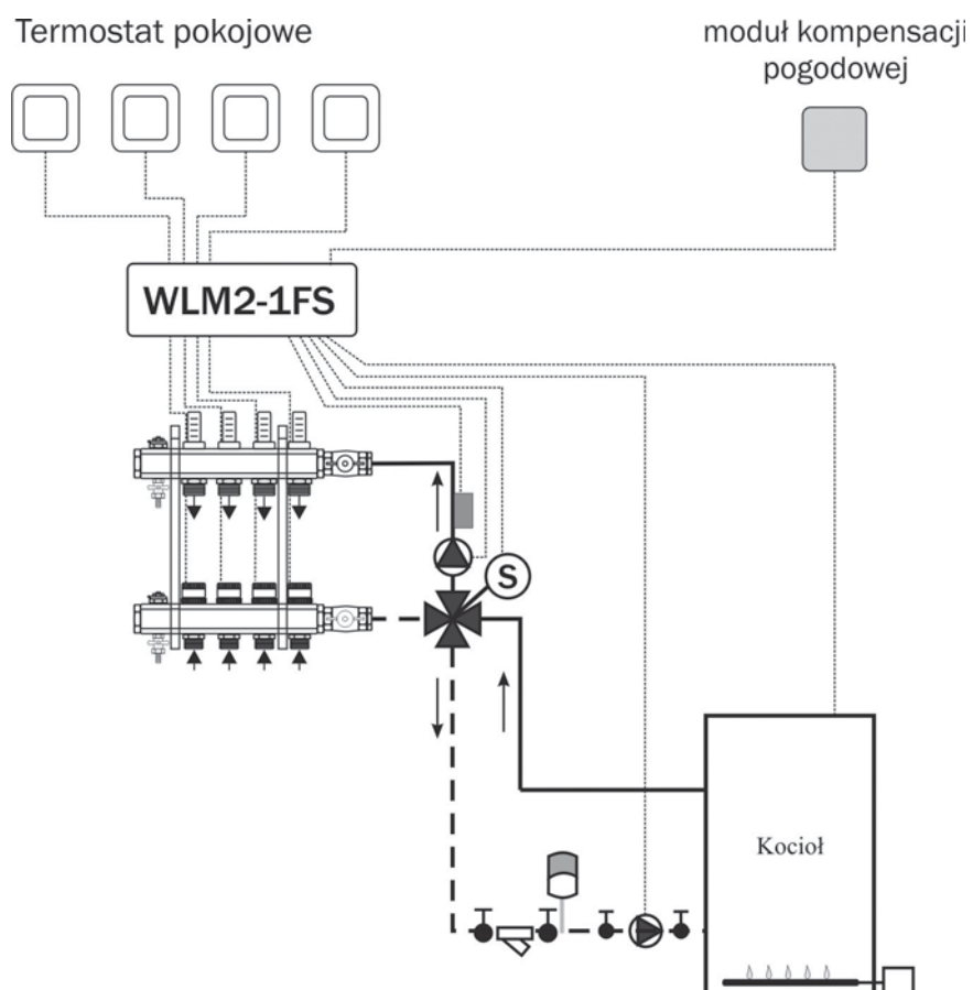
Sterowanie z wykorzystaniem kompensacji pogodowej z wykorzystaniem zaworu 4-drogowego
