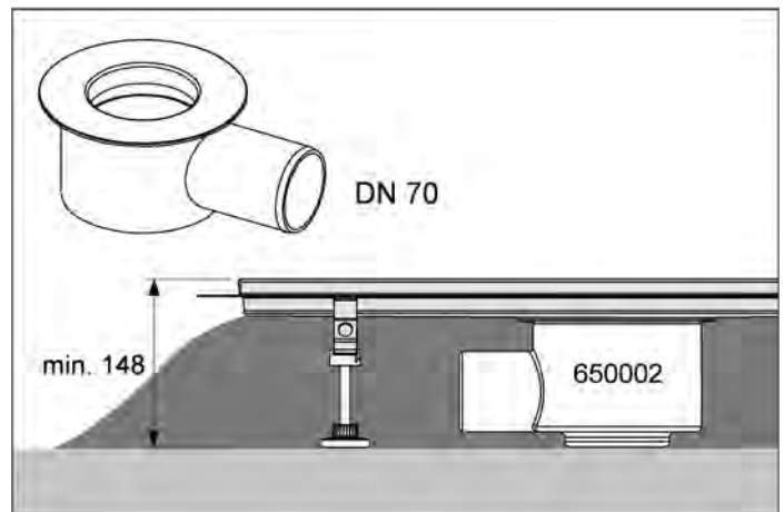
"Max" outlet
