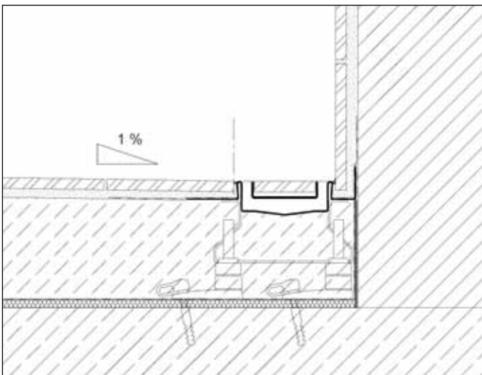
Einbau „Wandaufkantung“, Gefälle
