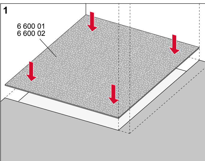
Optional: Schallschutzmatte Drainline zuschneiden und flächendeckend im Duschbereich positionieren.
