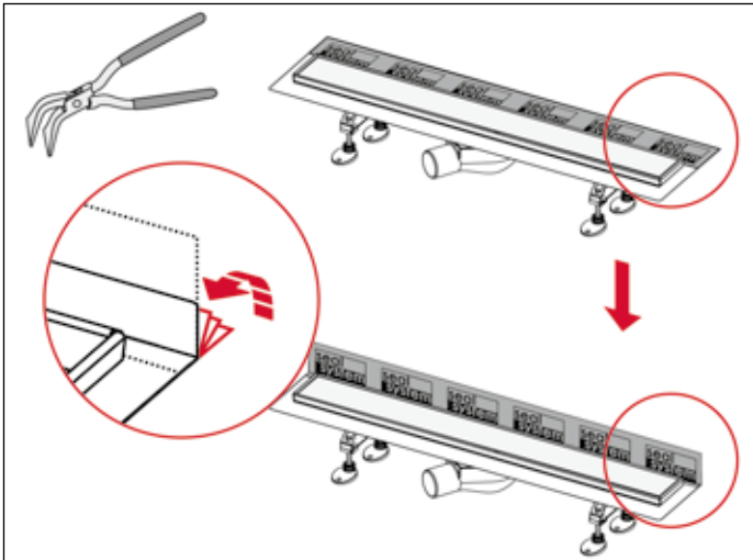
Abwinkeln des Rinnenflansches
