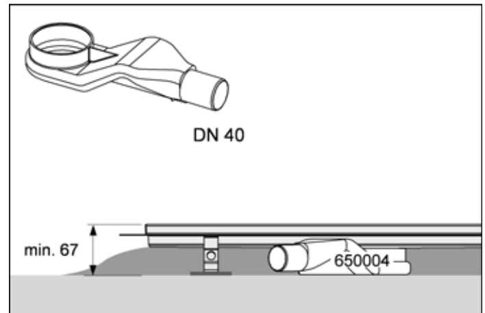
Ablauf „superflach“
