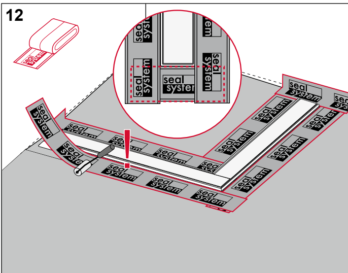
12 Seal System-Dichtband auf Länge schneiden, Schutzfolie entfernen und mit der dargestellten Überlappung auf Rinnenflansch und Estrich falten- und blasenfrei aufkleben und mit einem Roller andrücken.
