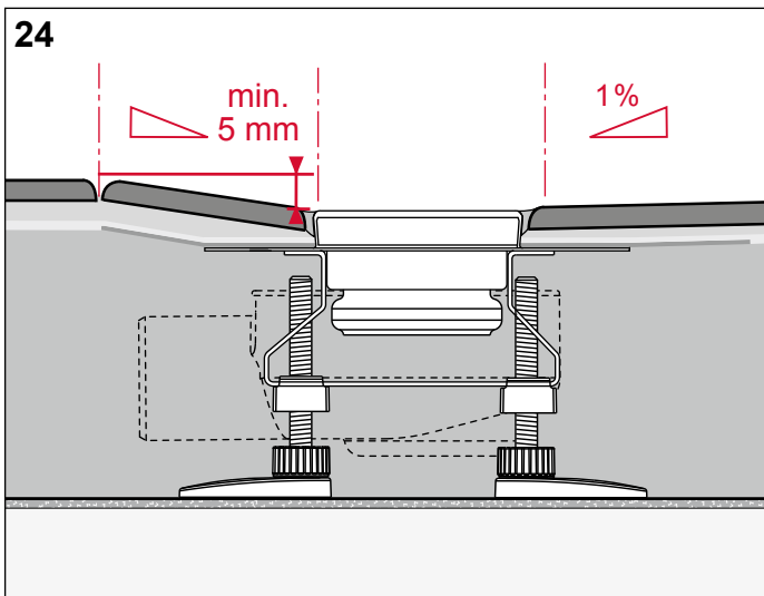
24 Gefälle und Gegengefälle prüfen.
