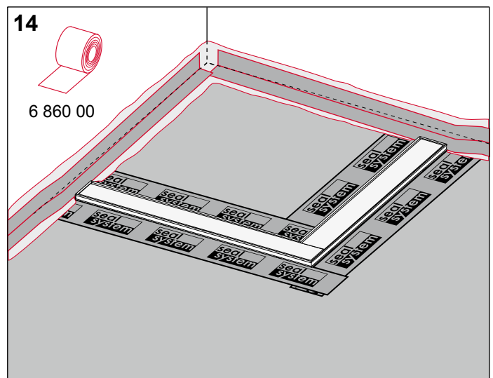
14 Direkt im Anschluss, in die frische Verbundabdichtung die Dichtbänder falten- und blasenfrei einlegen.
