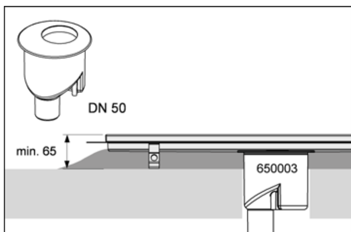
Ablauf „senkrecht“
