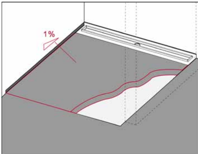
Gefälleausführung beim Einbau der Rinne an der Wand
