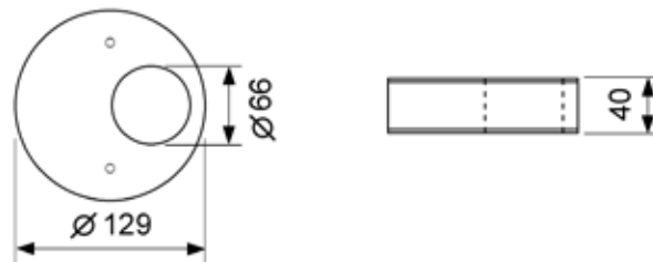
Abmessungen Brandschutzset
