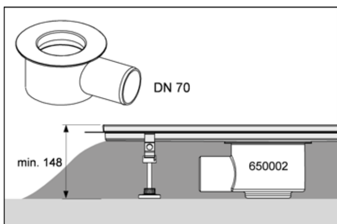
Ablauf „Max“
