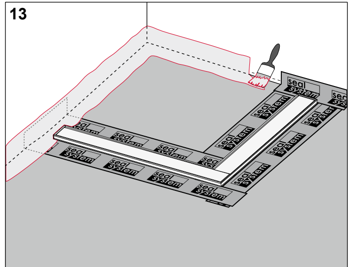
13 An den Übergängen von Wand und Estrich Verbundabdichtung auftragen. Bei Erstellung der Verbundabdichtung (Bild 13 bis 20) sind die Herstellerangaben zu beachten.
