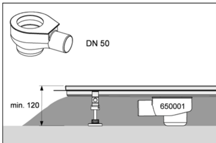
Ablauf „Norm“
