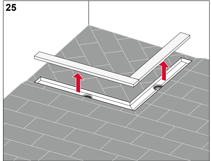
25 Rohbauschutz entfernen, Rinne säubern.
