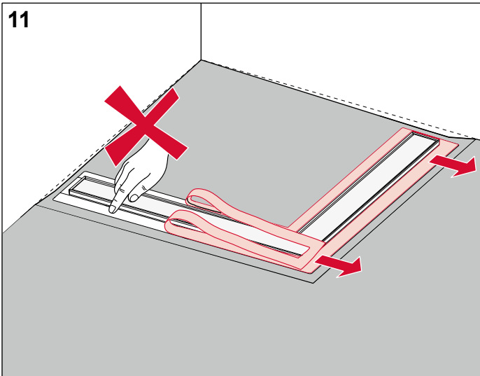
11 Schutzfolie vom Rinnenflansch vollständig abziehen. Flansch nicht mehr berühren, oder gar verschmutzen.
