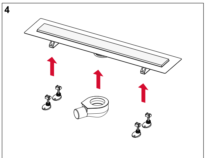
Ablauf montieren und ggfs. Montagefüße anclipsen.
