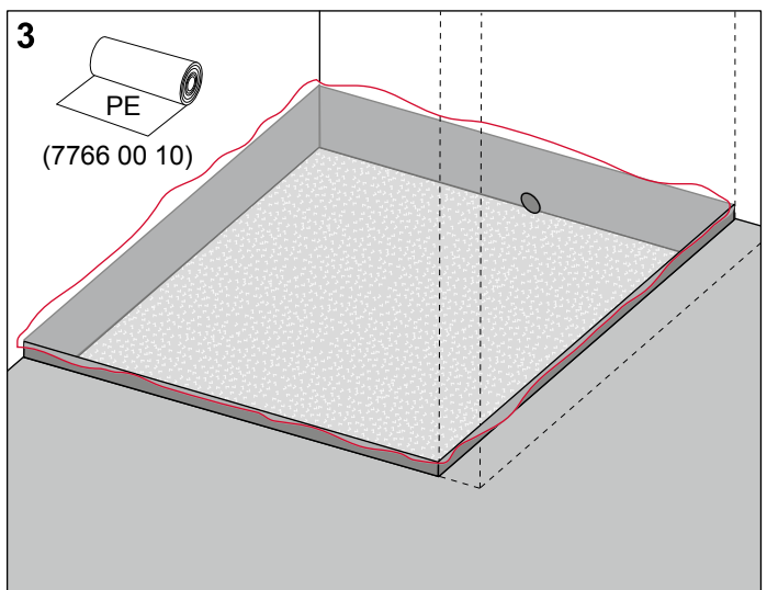
PE-Folie auslegen.
