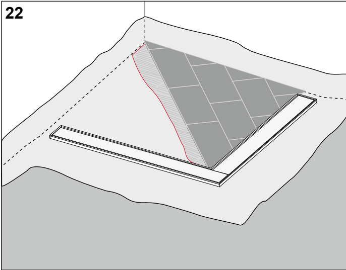
22 Bodenbelag (Fliesen o.ä.) aufbringen, dabei vorgeschriebenes Gefälle unbedingt einhalten.
