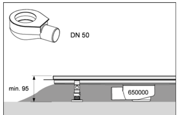
Ablauf „flach“
