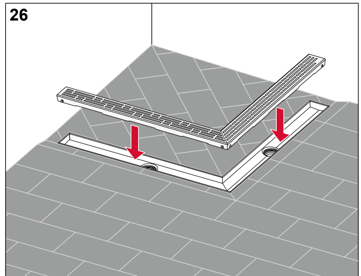
26 Gewünschte Abdeckung (Designrost, Fliesenmulde) einlegen.
