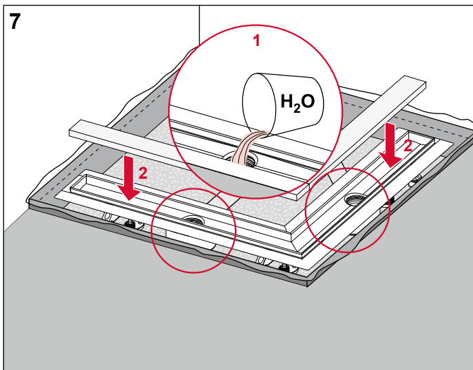
Rohbauschutz herausnehmen, Dichtigkeitstest durchführen und Rohbauschutz wieder einlegen.
