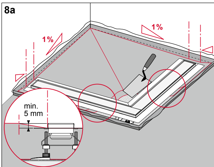
Estrich einbringen mit einem notwendigen Gefälle – im Duschbereich – von mind. einem Prozent zu beiden Schenkeln. Das Gegengefälle sollte mind. 5 mm betragen.
