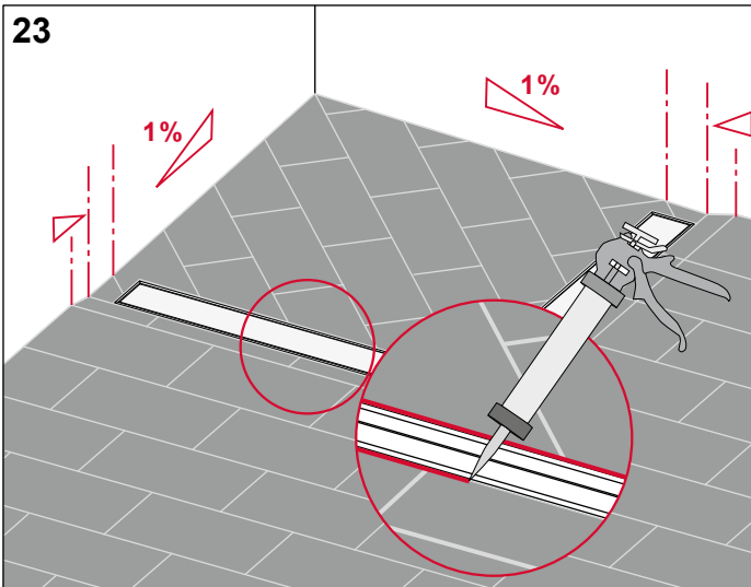
23 Fuge zwischen Edelstahlrinne und Fliese bzw. Naturstein mit dauerelastischem Material abdichten.
