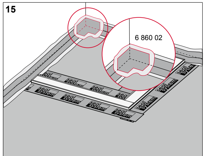
15 An Ecken Verbundabdichtung auftragen und die Dichtecken falten- und blasenfrei einlegen.
