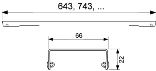
Abmessungen Designrost
