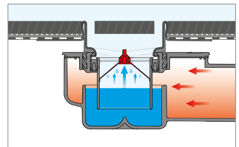
Schnitt TECEdrainline Membran-Geruchsverschluss.
