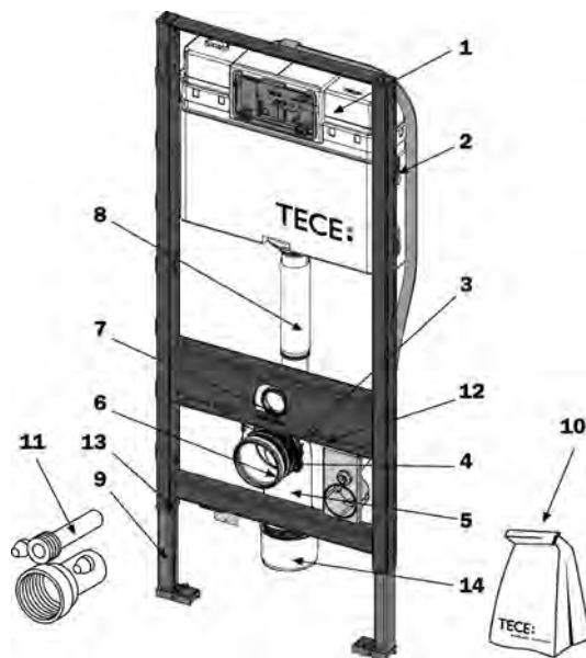
9300050 – WC-Modul für TOTO Neorest LE/SE Dusch-WC, Bauhöhe 1120 mm
