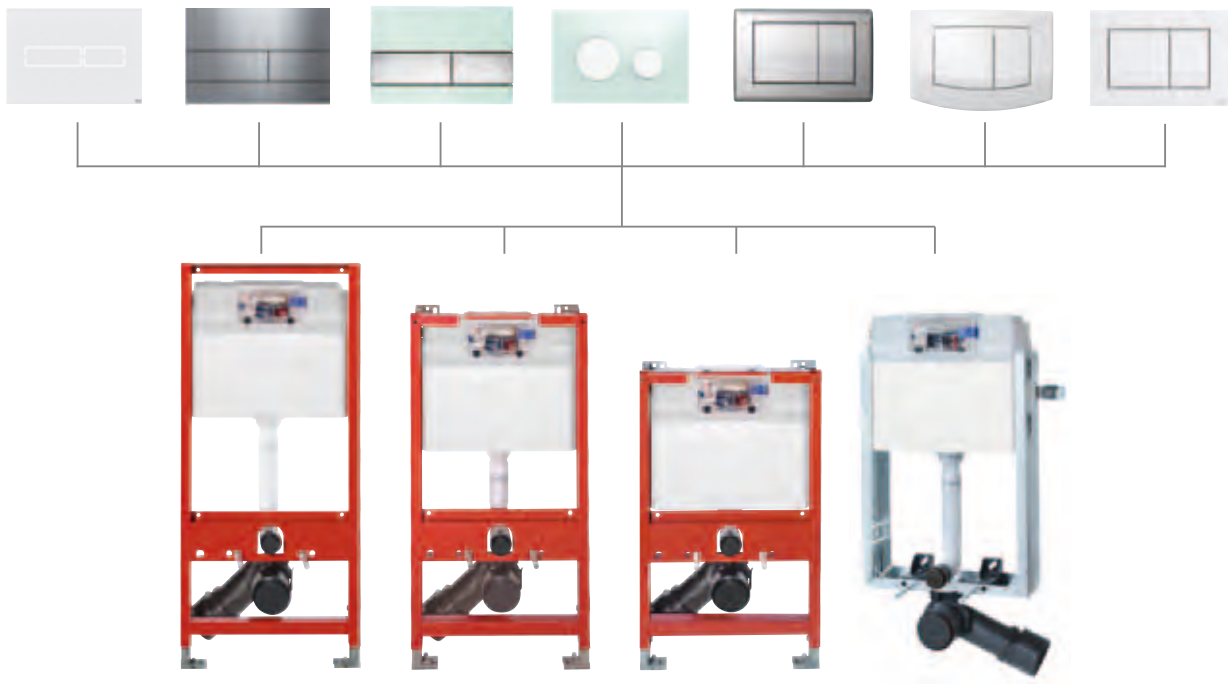
TECEprofil WC-Module und TECEbox Nassbauelement mit TECE-Spülkästen
