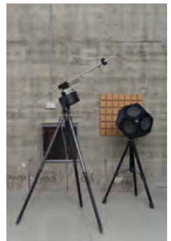
Abb. oben: Anlage zur Schallpegel- messung beim Fraunhofer Institut Stuttgart.
